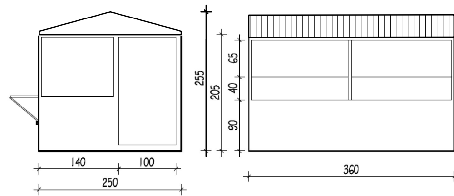
PROČELJE - PREDNJE
